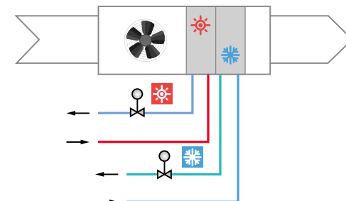
4-trubkový systém
