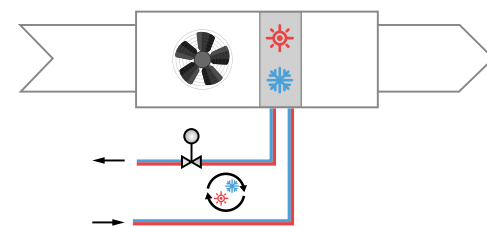
2-trubkový systém
